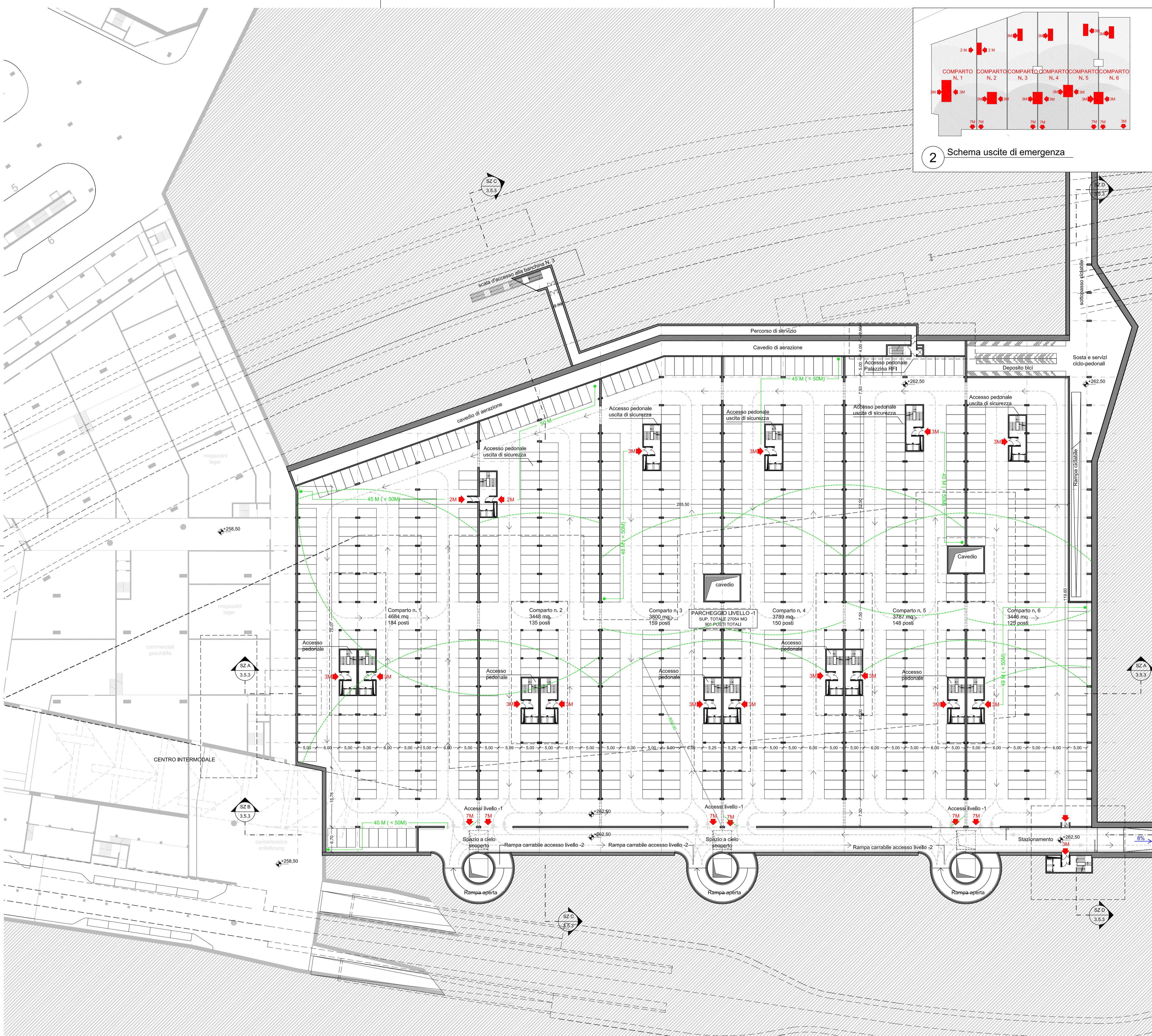
1 Pianta livello -1 - Grundriss Ebene -1 scala - masztab 1:500
