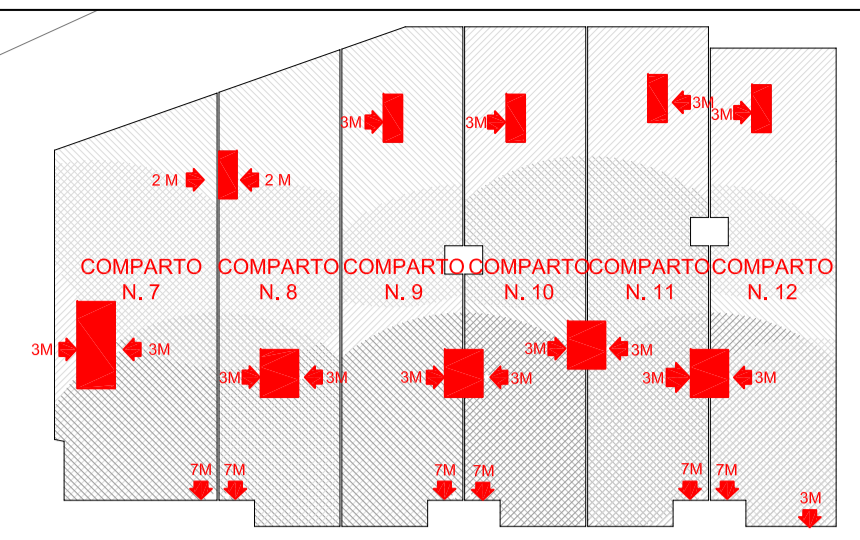
2 Schema uscite di emergenza
