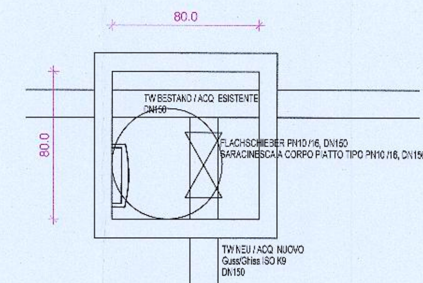
TRINKWASSERSCHACHT TW04 (SCHEMATISCH) POZZETTO ACQUA POTABILE TW04 (SCHEMATICO) M 1 : 20
