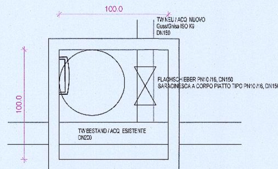
TRINKWASSERSCHACHT TW01 (SCHEMATISCH) POZZETTO ACQUA POTABILE TW01 (SCHEMATICO) M 1 : 20
