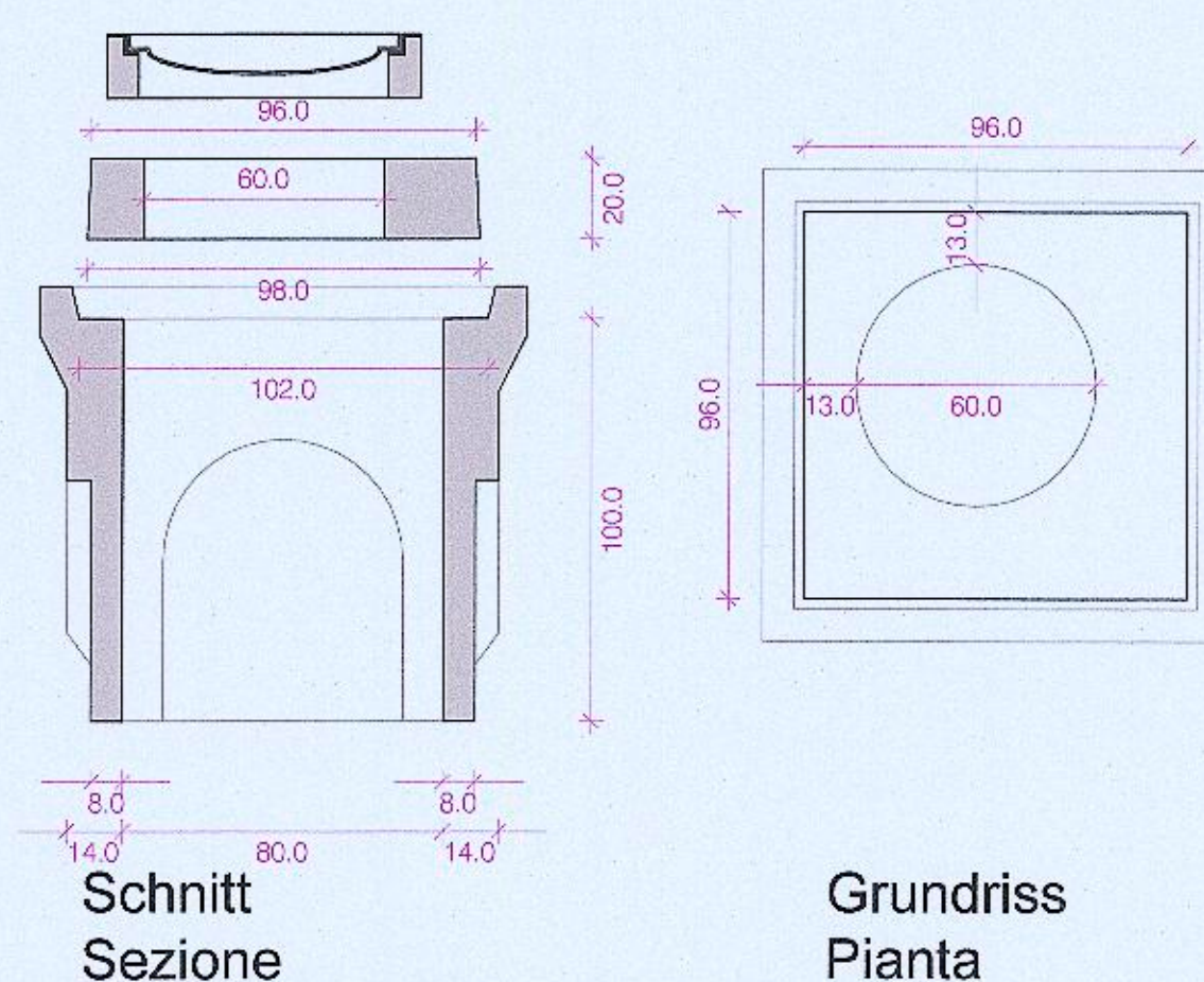
TRINKWASSERSCHACHT 80x80 POZZETTO ACQUA POTABILE 80x80 M 1 : 20
