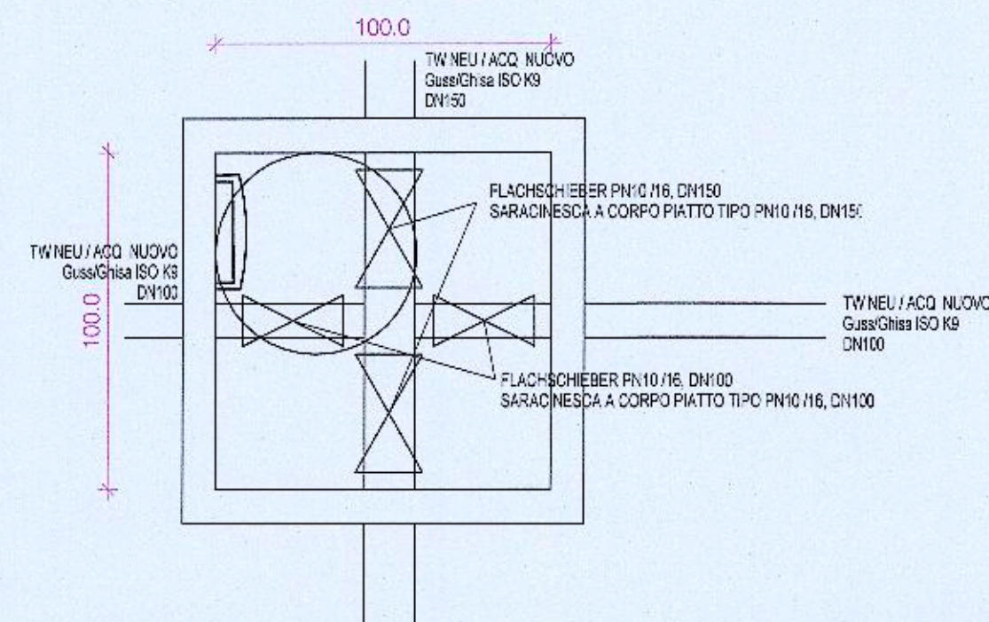
TRINKWASSERSCHACHT TW02 (SCHEMATISCH) POZZETTO ACQUA POTABILE TW02 (SCHEMATICO) M 1 : 20
