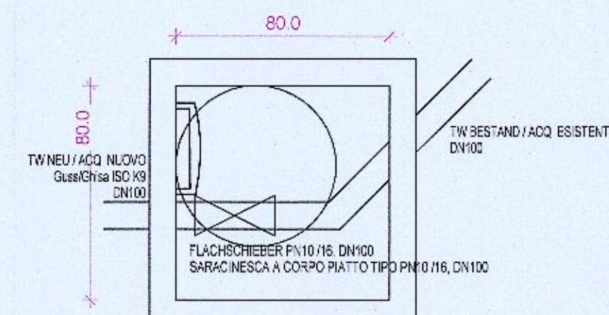
TRINKWASSERSCHACHT TW03 (SCHEMATISCH) POZZETTO ACQUA POTABILE TW03 (SCHEMATICO) M 1 : 20
