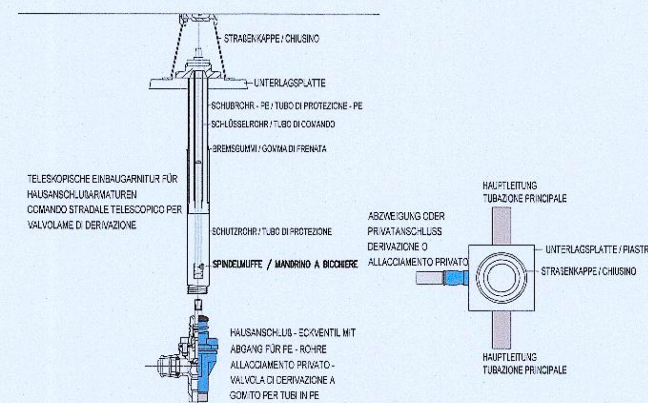
DETAIL HAUSANSCHLUSSSCHIEBER DETTAGLIO VALVOLUME DI DERIVAZIONE M 1 : 20
