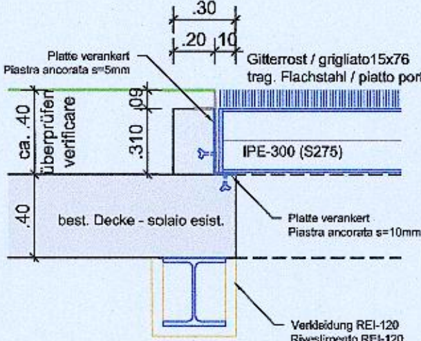
Schnitt / Sezione a-a Vertikalschnitt / Sezione verticale M 1:25
