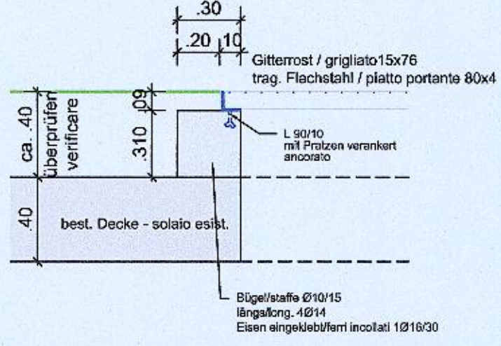
Schnitt / Sezione b-b Vertikalschnitt / Sezione verticale M 1:25
