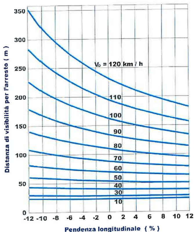
DIAGRAMMA DISTANZE DI VISIBILITA' PER L'ARRESTO
