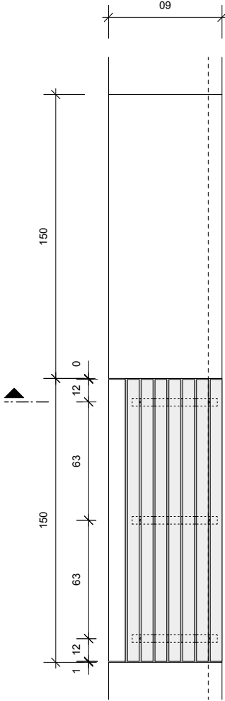
Aufsicht M 1:20
