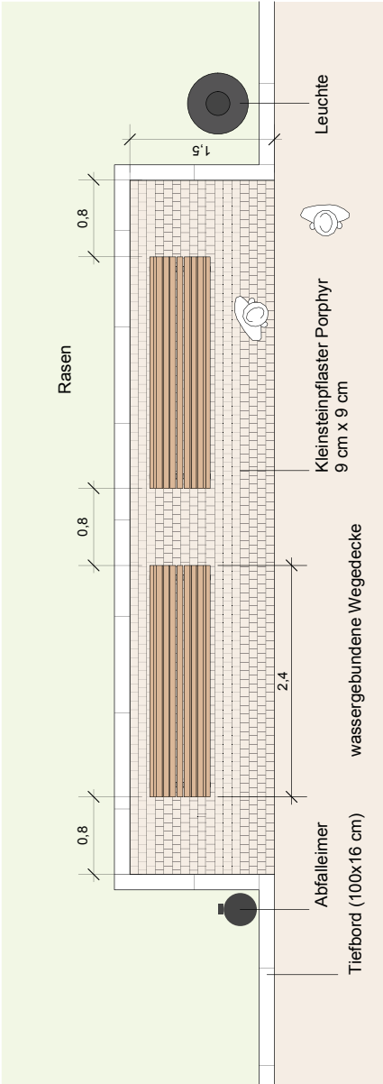
Aufsicht M 1:50
