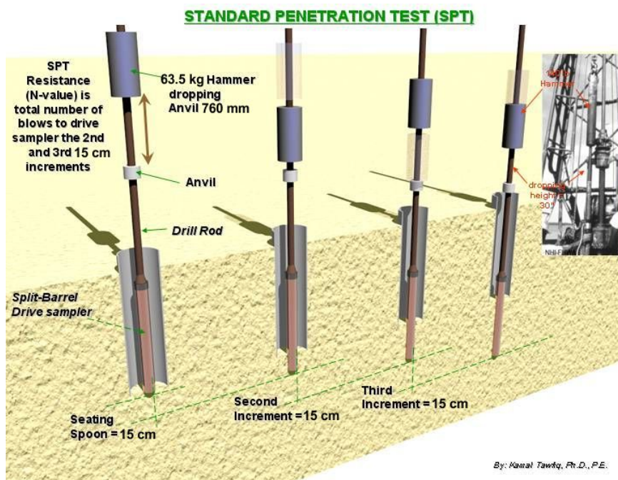
Figura 9 – Schema prova S.P.T.
