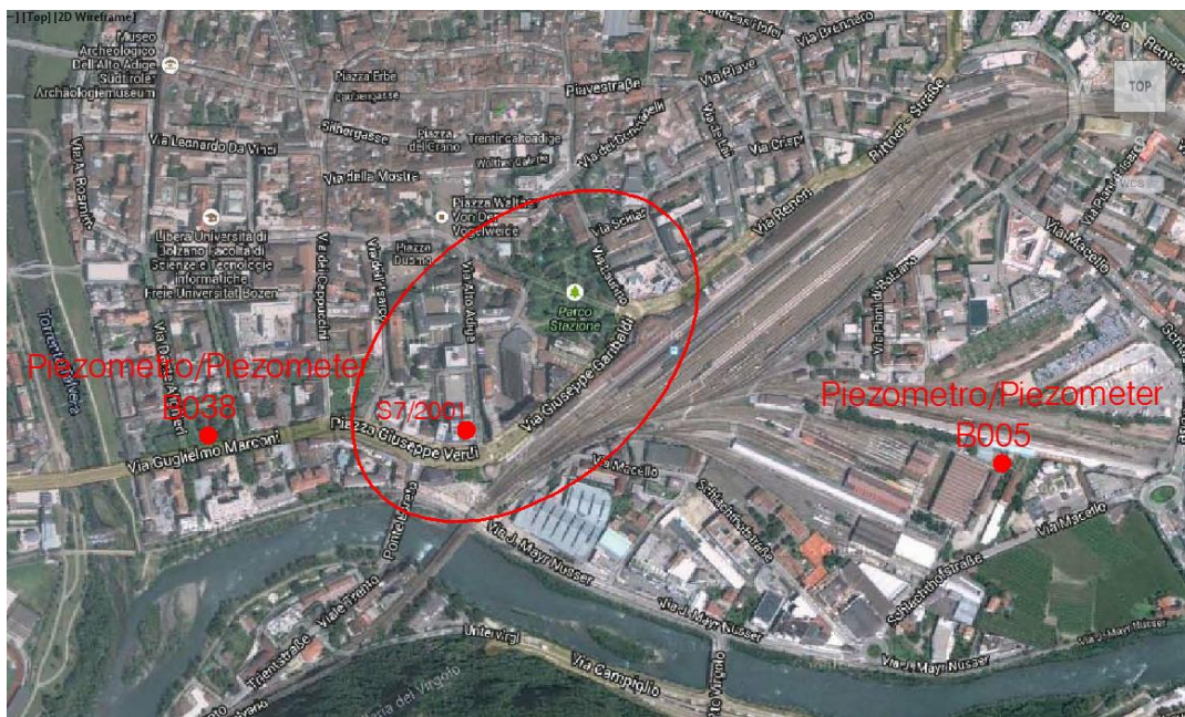
Figura 3 – Ubicazione dei piezometri esistenti nei pressi del sedime
