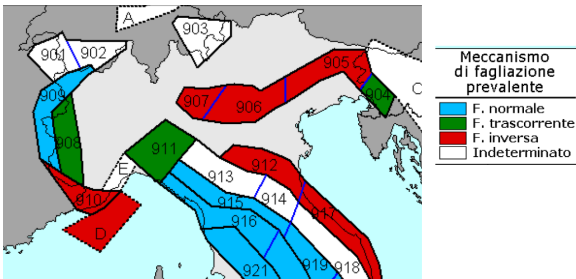
Figura 9a - Meccanismo di fagliazione prevalente atteso per le diverse zone sismogenetiche riconosciute (Fonte INGV)
