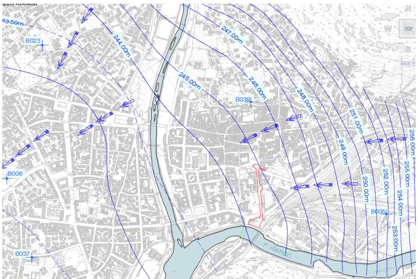
Figura 5a – Ricostruzione della piezometria della falda a superficie libera, misurata nel luglio/agosto 1997
