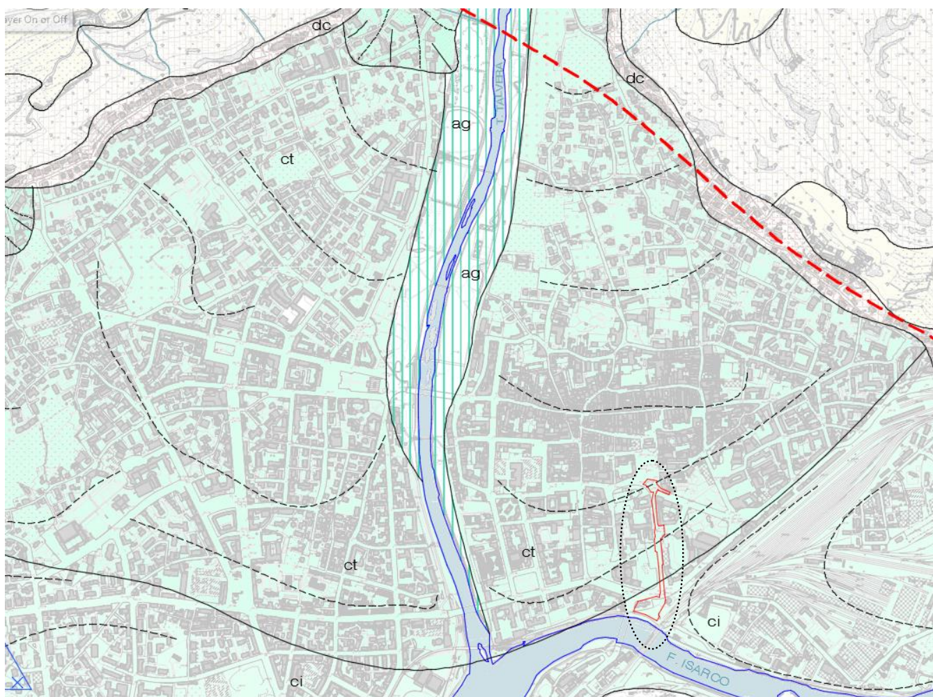
Figura 2b – Carta geomorfologica di Bolzano -
